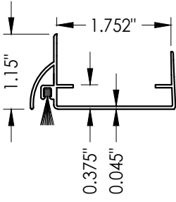
45 DOOR SWEEP
